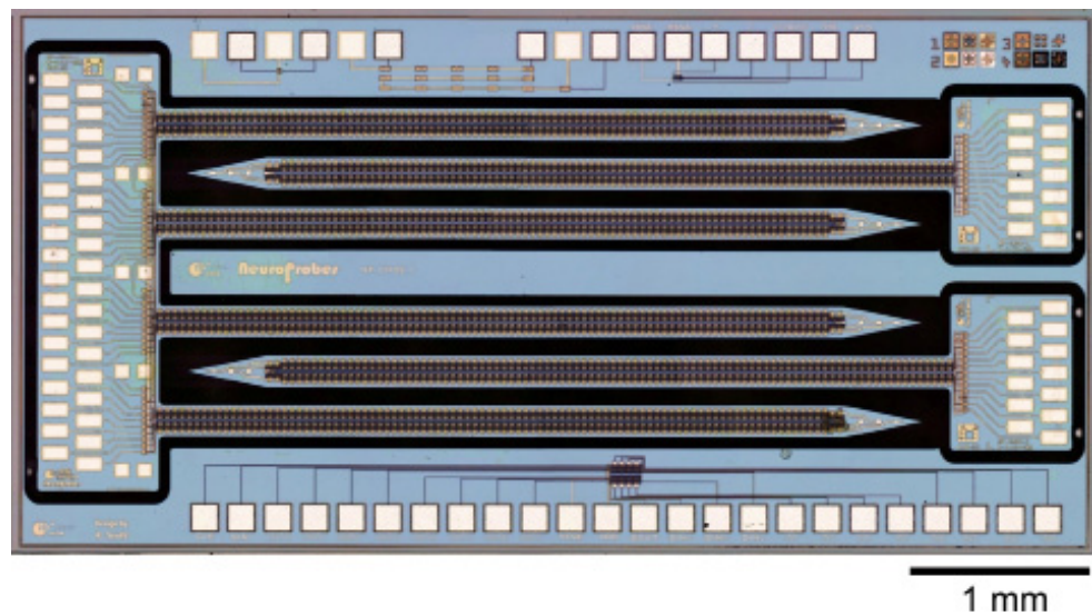
Hochdichte CMOS-basierte Elektrodenarrays für die elektrische Tiefenkontrolle
