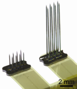
3D-Mikronadelarray
